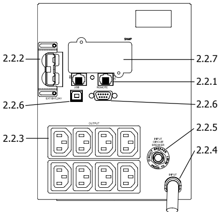
SXL-1000A LCD
